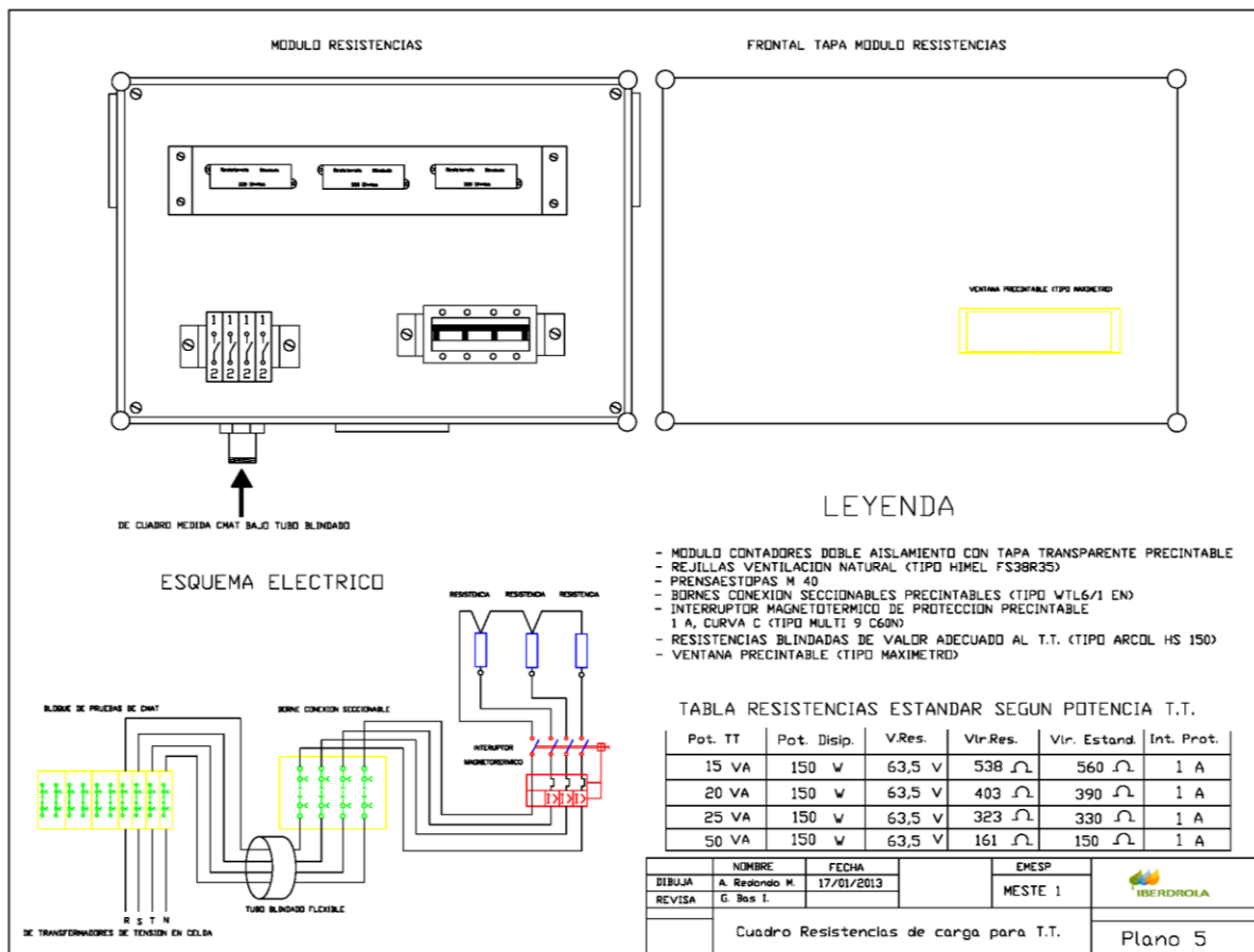
Módulo, esquema y fotos ilustrativas caja resistencia de cargas
